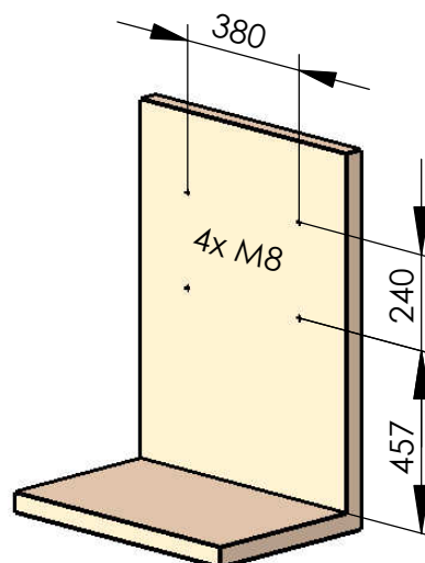
empfohlenes Lochbild
